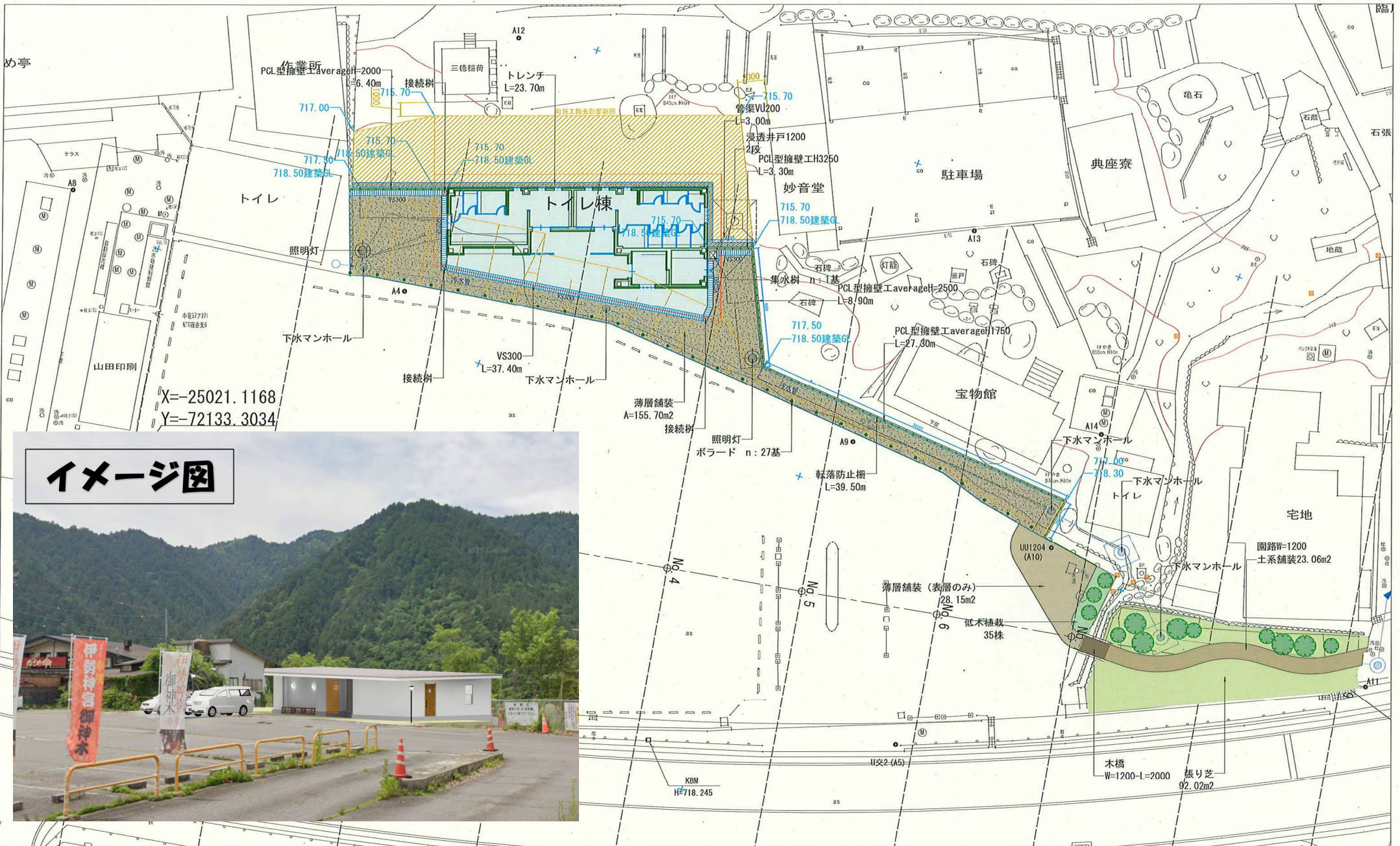
寝覚の床観光拠点整備計画平面図
